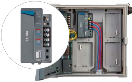
Módulo de salida para decodificadores EZ-DM y programadores ICC2 y HCC Altura: 115 mm Anchura: 64 mm Profundidad: 42 mm
