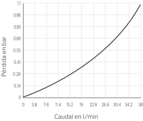
FLEXSG Y PÉRDIDA POR FRICCIÓN DE CODO ARTICULADO
