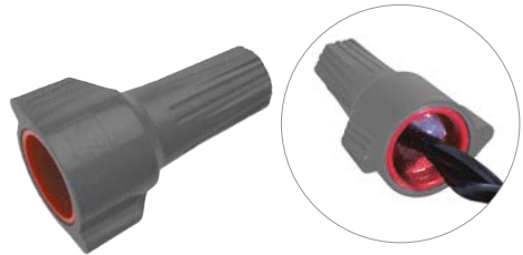
Conector de cables estanco Altura: 3,5 cm Cable mínimo: 3 de 0,8 mm² Cable máximo: 2 de 6 mm² con 1 de 3 mm²
