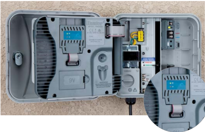
PROGRAMADOR P2C-400 CON MÓDULO PC-WIFI CONECTADO
