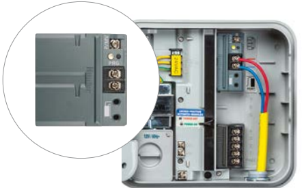
Módulo de salida del decodificador PC-DM para programadores Pro-C y HPC Altura: 76 mm Anchura: 76 mm Profundidad: 32 mm
