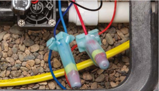
KIT DE CONECTOR ESTANCO DBRY-6
