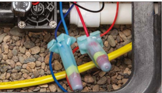
KIT D'ÉPISSURE ÉTANCHE DBRY-6
