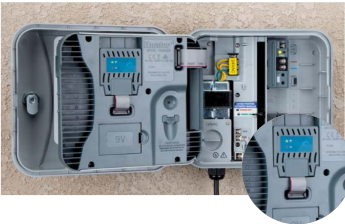
PROGRAMMATEUR P2C-400 AVEC MODULE PC-WIFI CONNECTÉ
