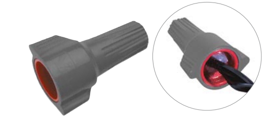
Capuchon de connexion étanche Hauteur : 3,5 cm Taille de câble minimum : 3 câbles de 0,8 mm² Taille de câble maximum : 2 câbles de 6 mm² avec 1 câble de 3 mm²
