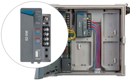
Module de sortie du décodeur EZ-DM pour les programmeurs ICC2 et HCC Hauteur : 115 mm Largeur : 64 mm Profondeur : 42 mm
