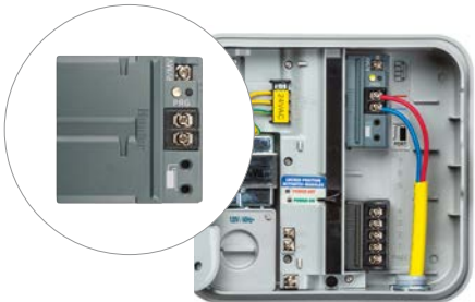
Module de sortie du décodeur PC-DM pour les programmeurs Pro-C et HPC Hauteur : 76 mm Largeur : 76 mm Profondeur : 32 mm
